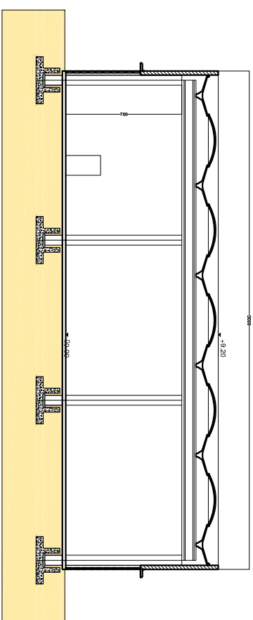
SEZIONE A-A
